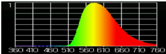
一般直管LED照明 スペクトル
