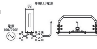
【接続図】
