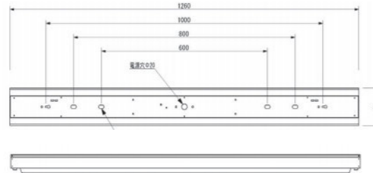
【仕様図】
