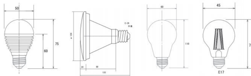
【仕様図】
