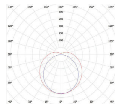
蛍光灯代替LED配光曲線
