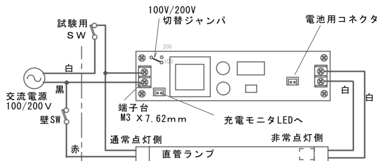
【配線図】
