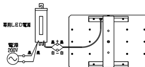
【結線図】
